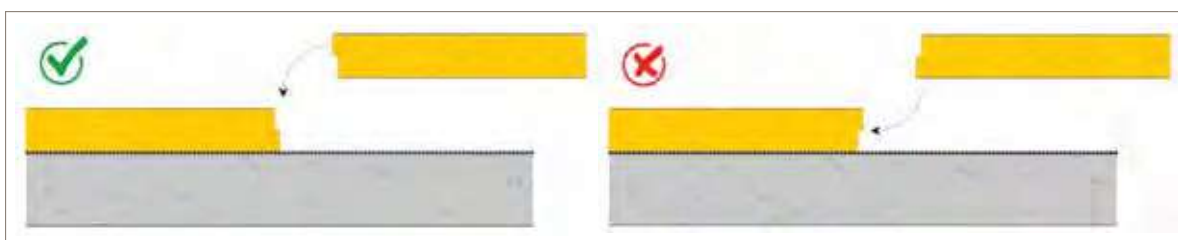
Afbeelding 28: Montage van isolatieplaten met spinning (links: correcte toepassing, rechts: foutieve toepassing)
