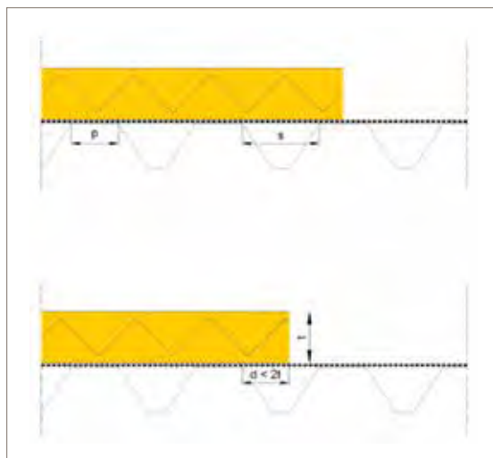
Afbeelding 21: Aanbrengen van isolatieplaten op een stalen ondergrond (Boven: aanbevolen montage - ondersteunde randen; Onder: Beperking van uitkraging voor t \geq 50 mm)
