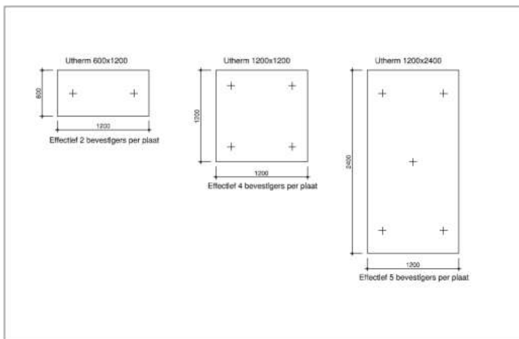
Figuur 3b – Bevestigingspatronen (minimaal aantal bevestigings) voor niPIR-N
